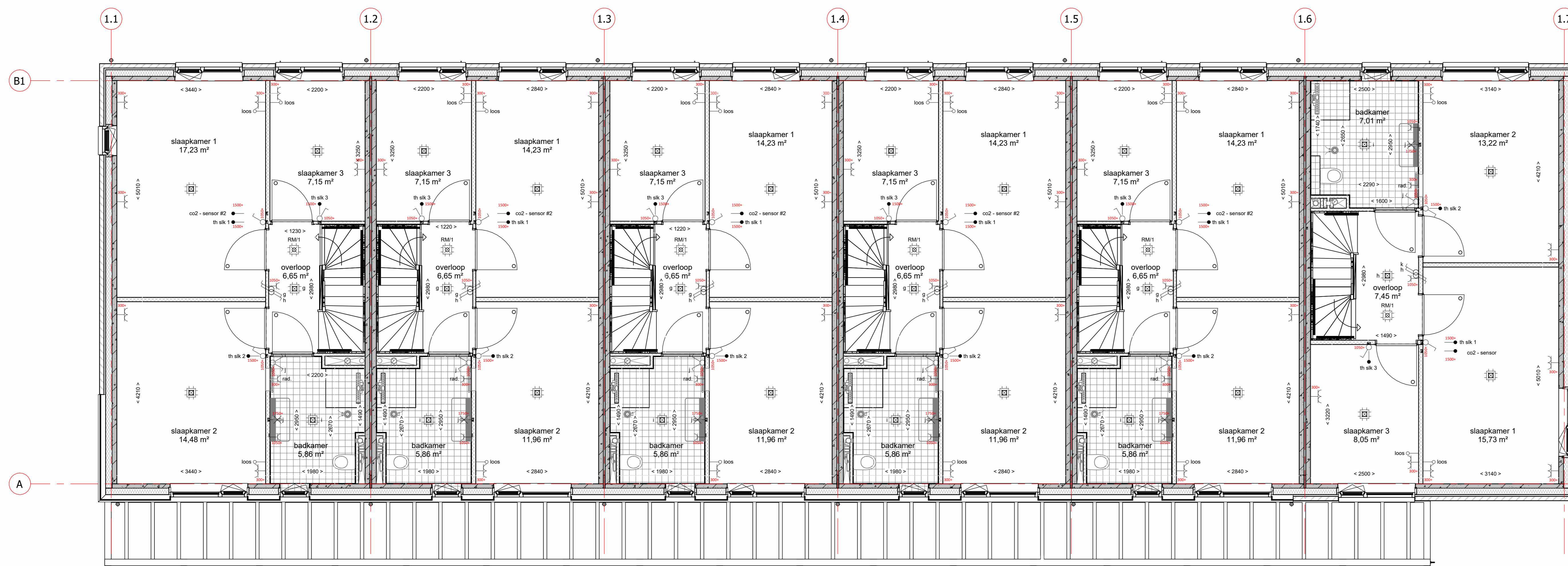
1e verdieping schaal 1:50
