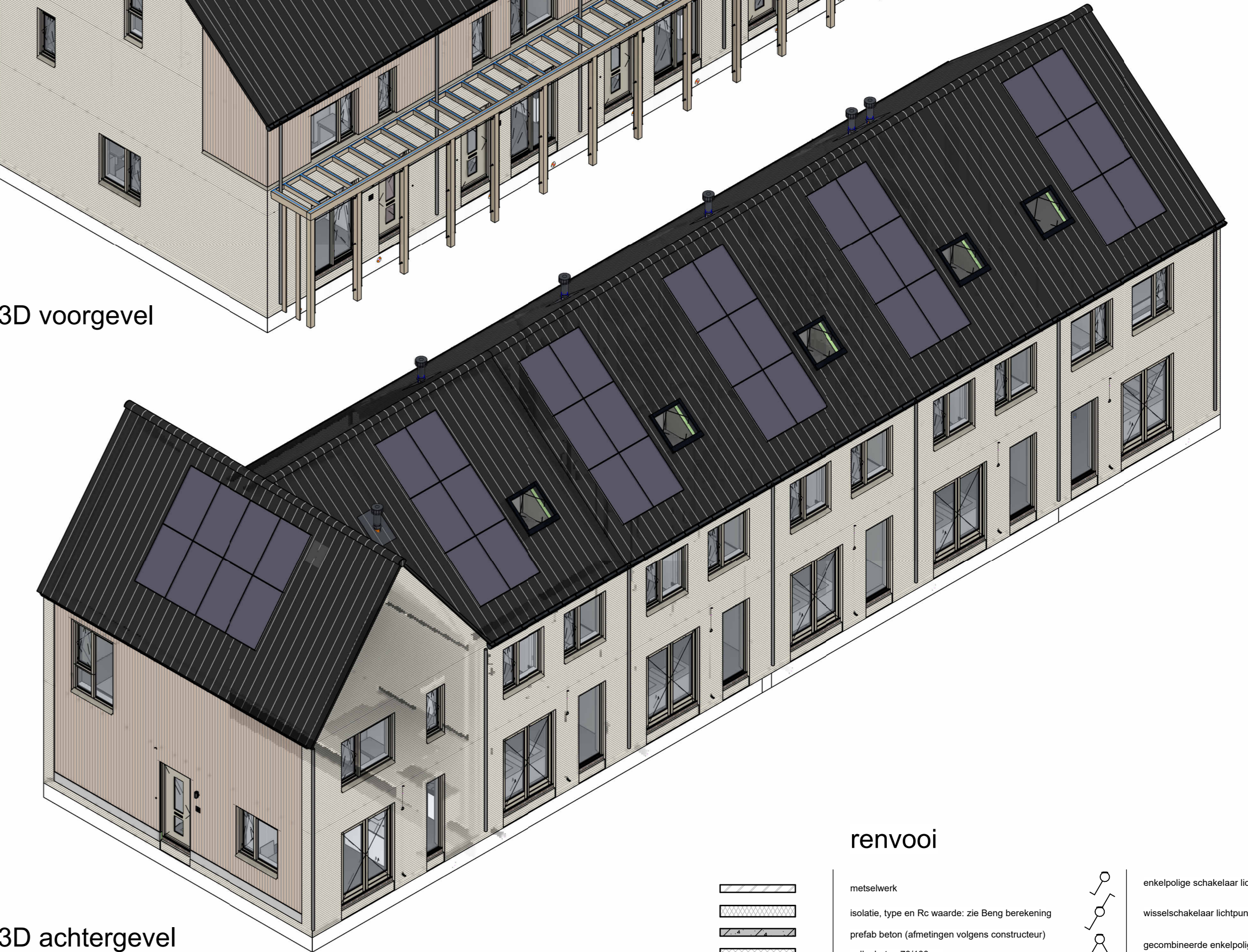
3D achtergevel
