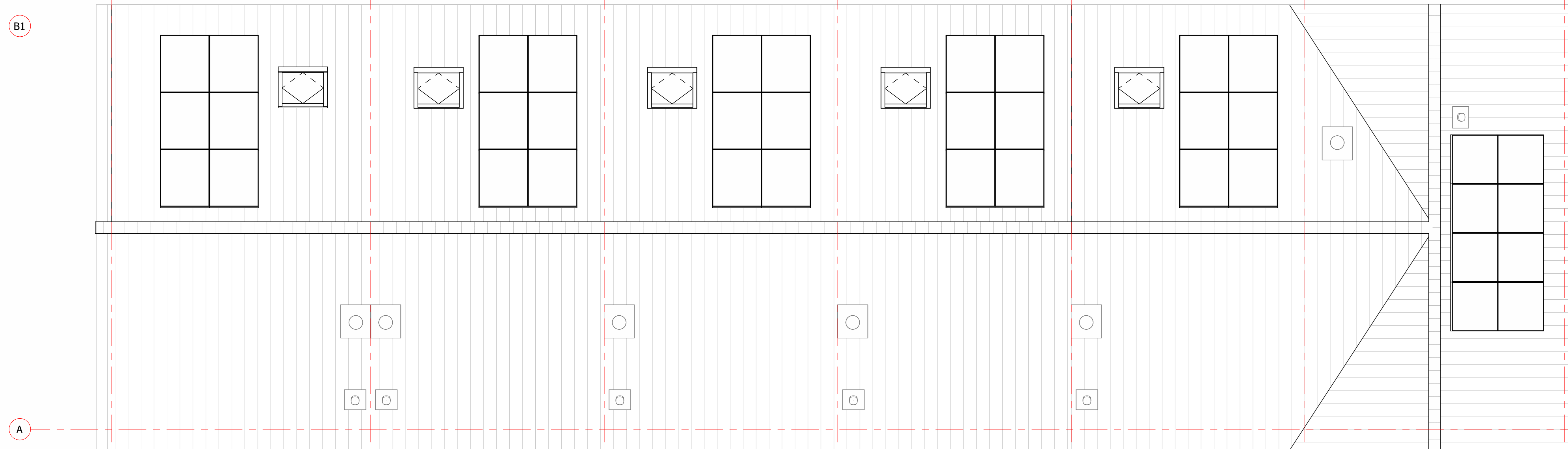
dakoverzicht schaal 1:50
