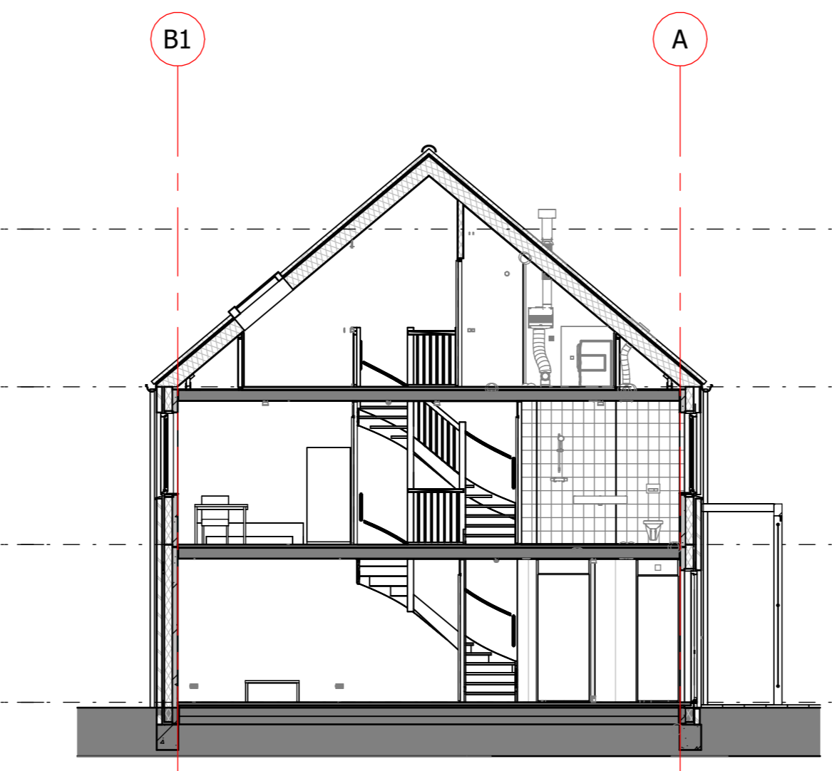
langsdoorsnede bnr 01 schaal 1 : 100
