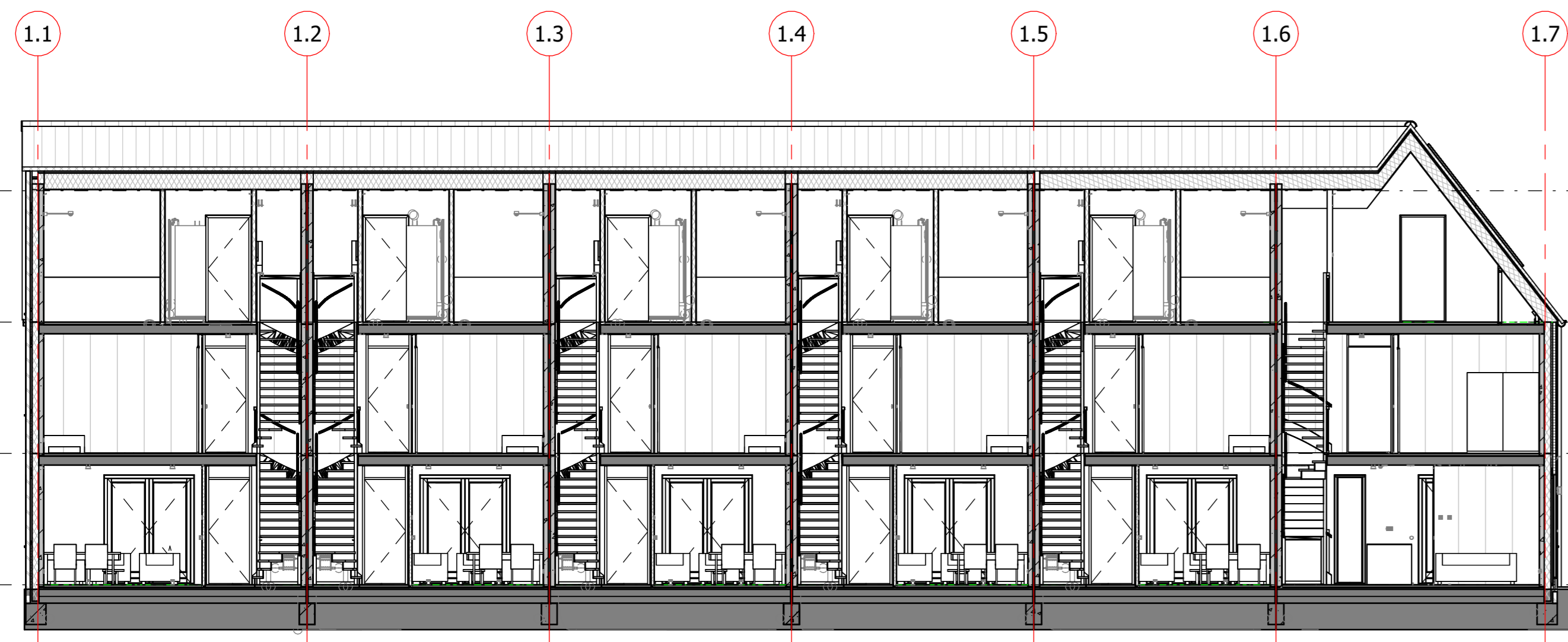
dwarsdoorsnede schaal 1 : 100
