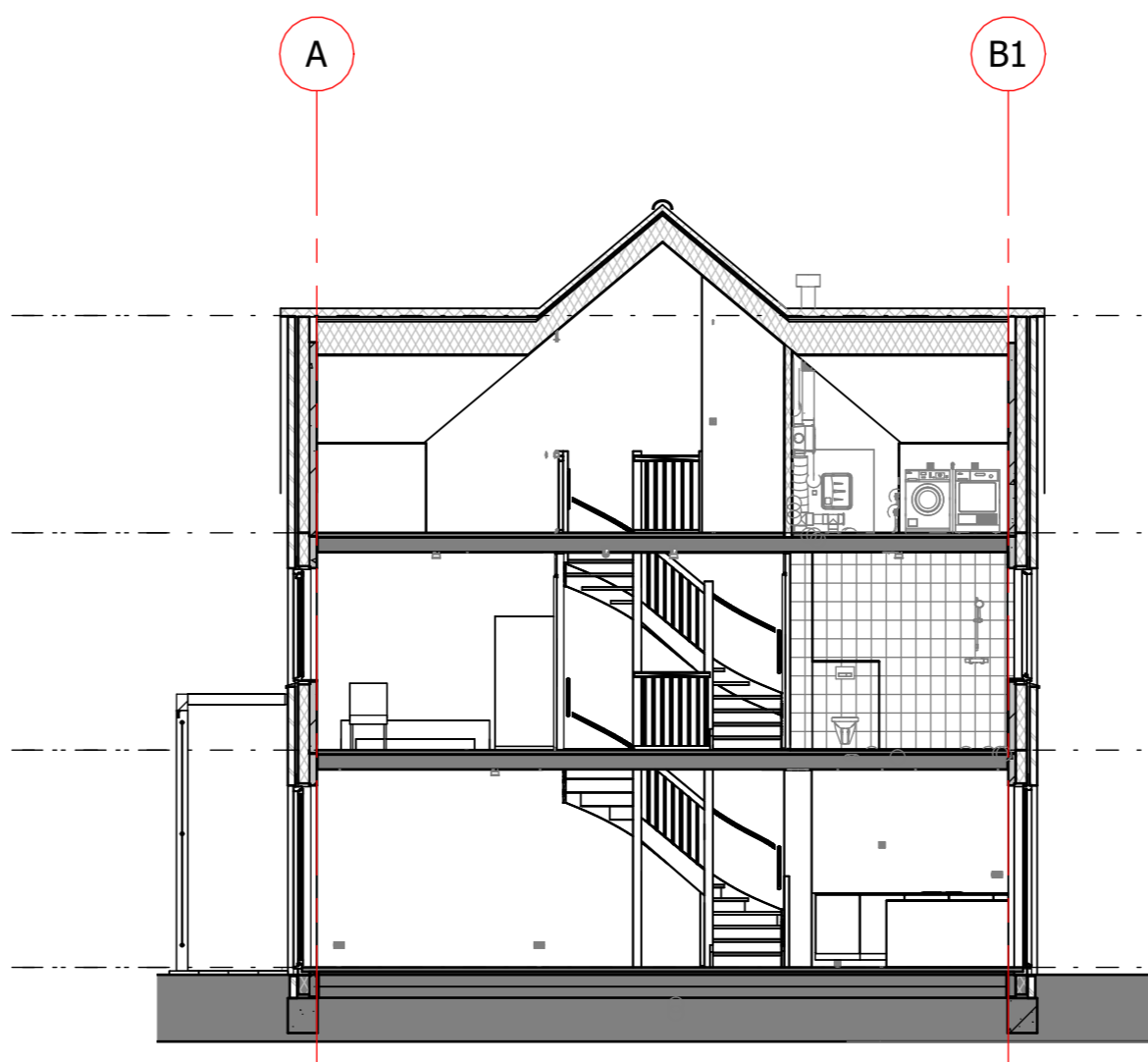
langsdoorsnede bnr 06 schaal 1 : 100
